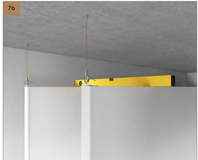
7b Plasser et vater på toppen eller under baflene for å sikre at de henger jevnt og er i vater i alle retninger. Nivellering gjøres ved å løsne wirelåsen på kroken og justere med wiren.
